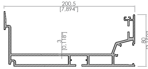
Dere Profil Gutter Profile
