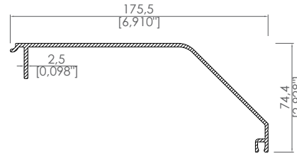
Motor Kutusu Kapağı Motor Box Cover
