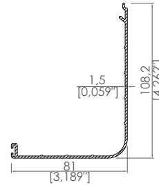
Motor Kutusu Kapagı Profili Motor Box Cover Profile
